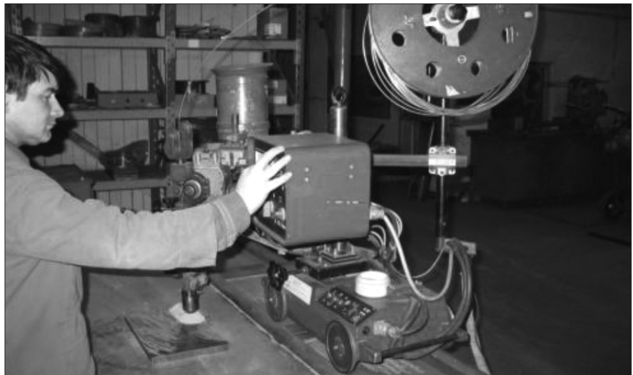
Varjenje pod praškom v varilnici
